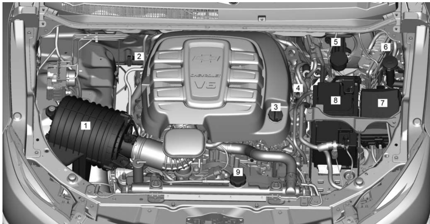
Бензиновый двигатель V6, 3.6L, VVT
