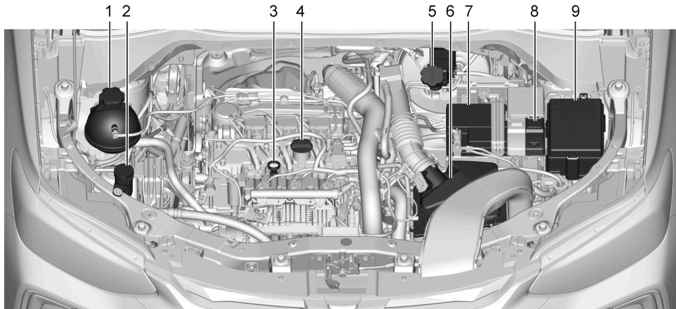
Dvigatel bo'linmasi umumiy ko'rinishi
